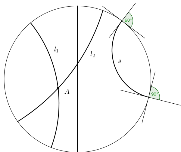
Kuva 2: Poincarén kiekko.
