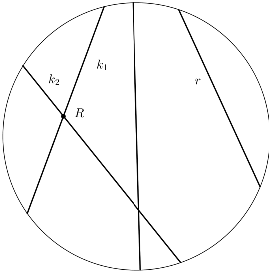
Kuva 5: Kleinin kiekko.
