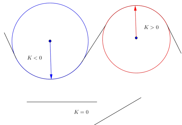
Kuva 7: Käyrän kaarevuus.
