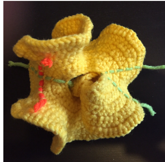
Kuva 1: Esimerkki hyperbolisesta pinnasta.
